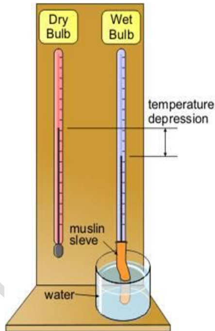
الشكل (1): الأجهزة والأدوات اللازمة لقياس الرطوبة النسبية.
